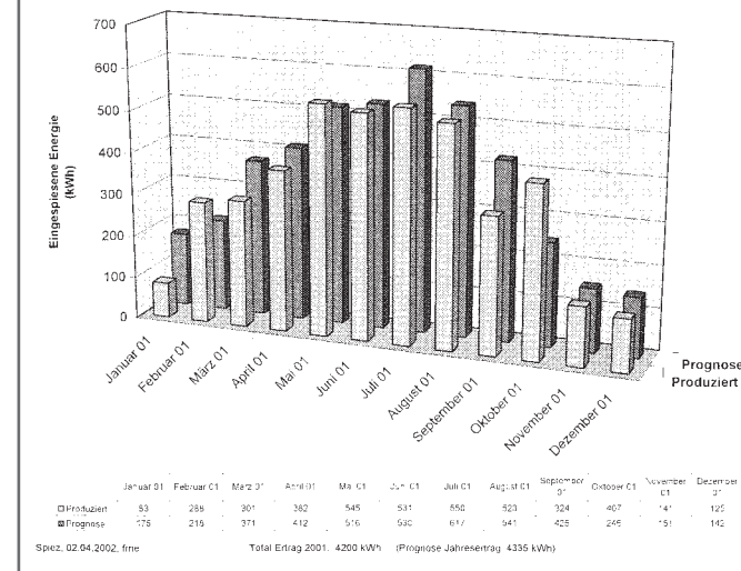
Prognose und Ertrag der 4,3 kWp Fotovoltaikanlage Längenstein
