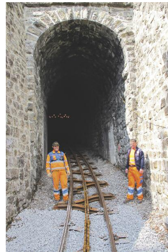
Im «Härdtunäl» wird es sehr eng! Gut erkennbar sind die neuen Doppelzahnstangen sowie die stabileren Ypsilon-Schwellen.
