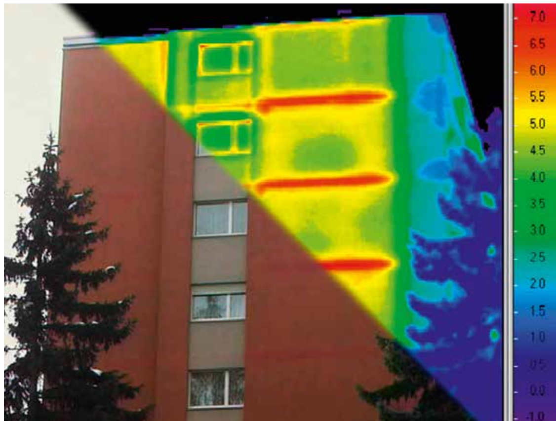
Kombiniertes Sichtbild/Wärmebild mit Temperaturskala eines Mehrfamilienhauses.
