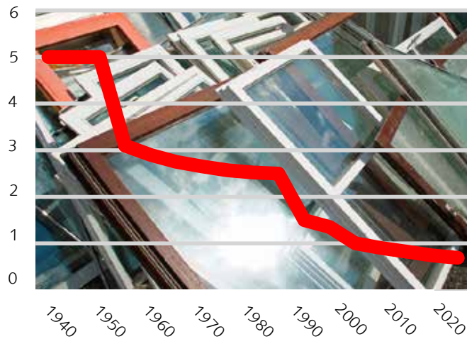
Entwicklung Dämmwert Fenster Uw-Wert in W/m²K.
