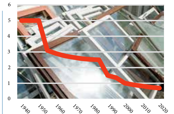
Entwicklung Dämmwert Fenster Uw-Wert in W/m²K (Bild: pixelio.de)
