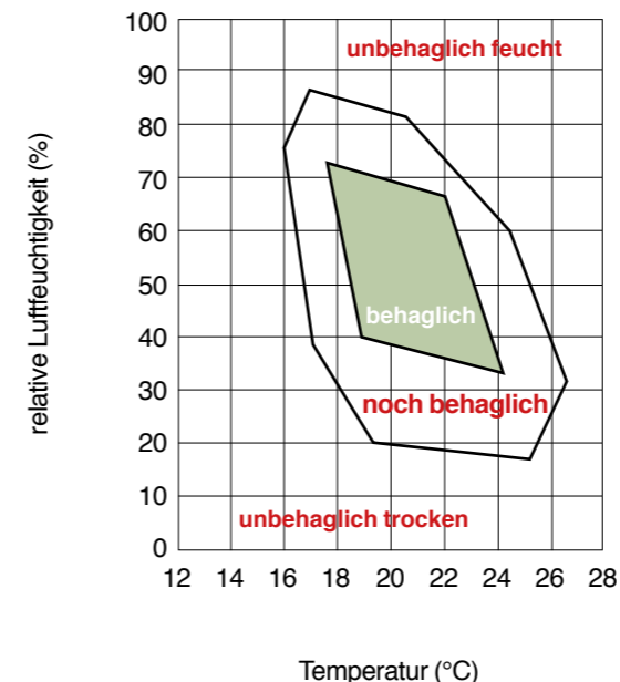
Behaglichkeitsbereich (Quelle: Wegweiser für eine gesunde Raumluft)
